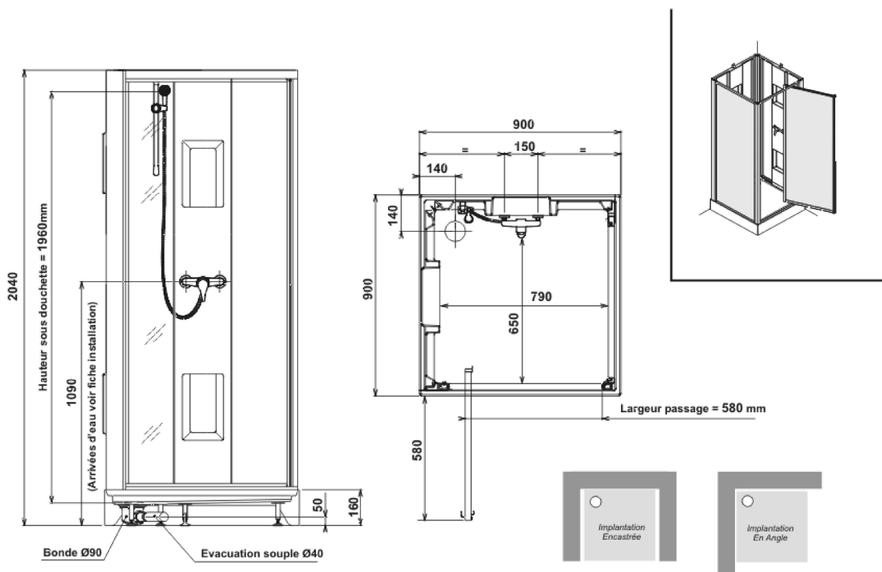
Leda ENCOMBREMENTS - L11IZ889 CABINE IZI BOX CARRE 90 PORTE PIVOTANTE
