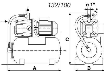
AQUAJET 102/20-60-80 132/100
